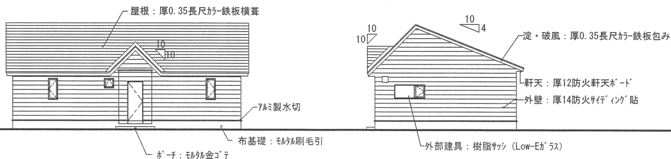
立面図 S=1/200
