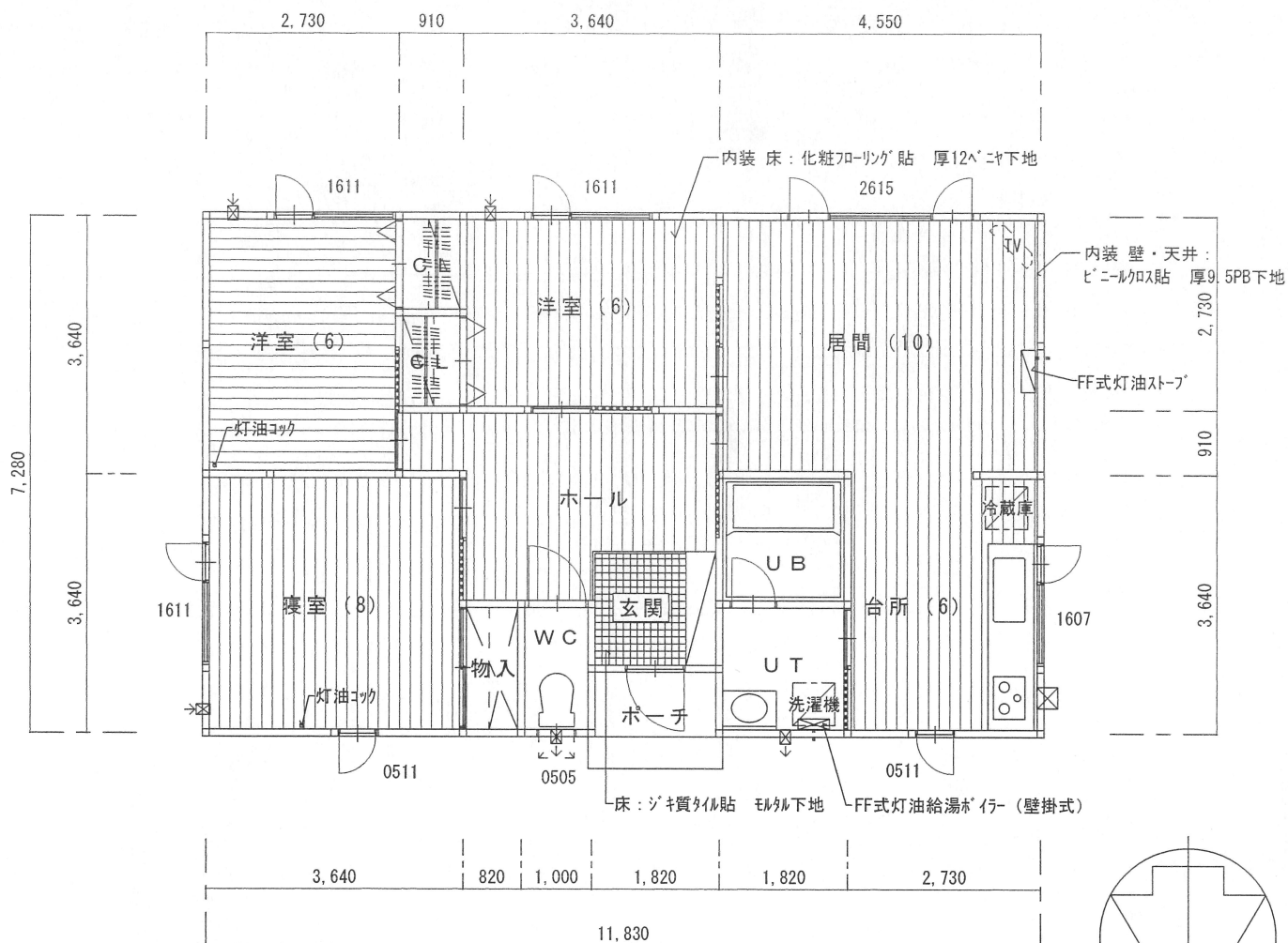
平面図 S=1/100
